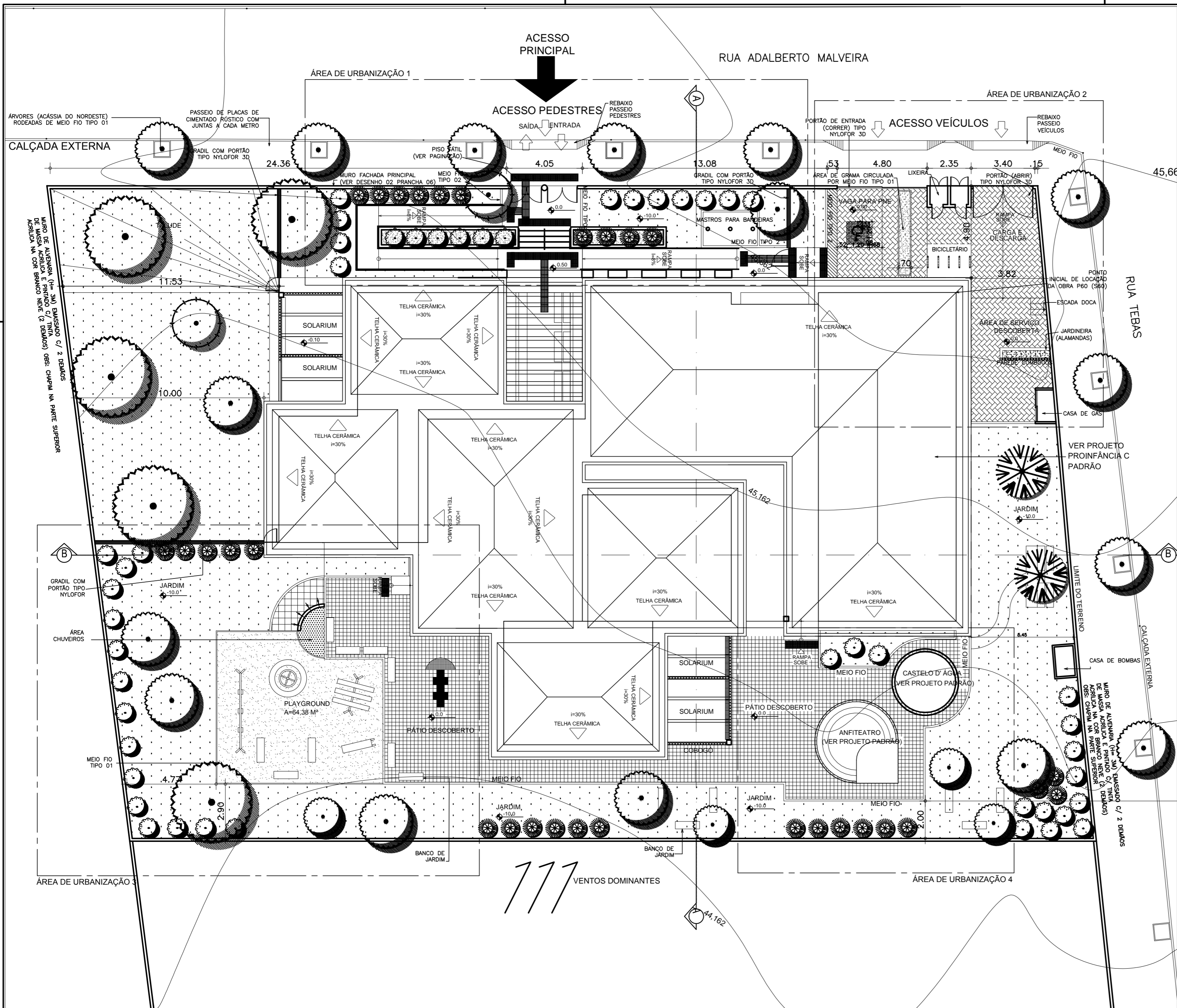
1 PLANTA DE LOCAÇÃO / URBANIZAÇÃO ESC.: 1:150
